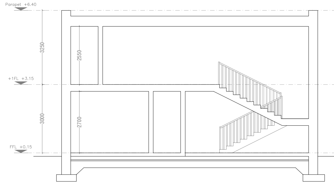
Creche Section A.A
